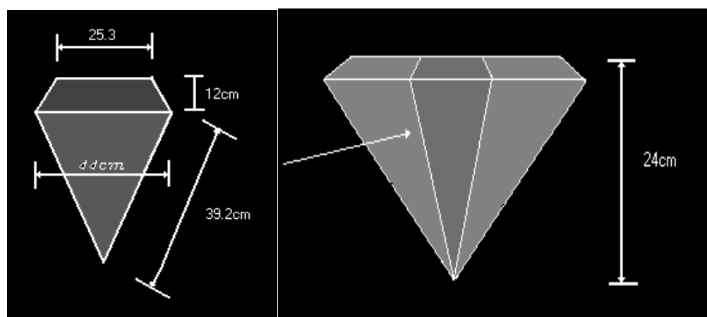
Figura 3. Diseño de las bases laterales internas de la estufa solar.
