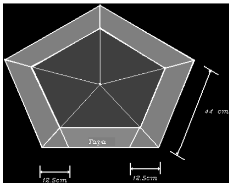
Figura 4. Diseño de la parte superior externa de la estufa solar.
