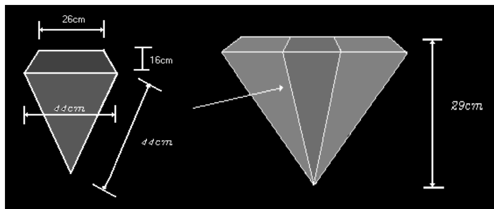
Figura 2. Diseño de las bases laterales externas de la estufa solar.
