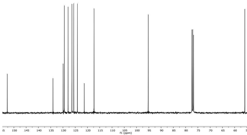
Espectro 2. Espectro de RMN 13 C (CDCl 3 ) de molécula 2.
