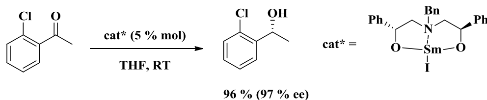
Esquema 17. Reducción de cetonas aromáticas de Evans.
