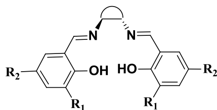
Esquema 20. Estructura general de ligante tipo Salen .
