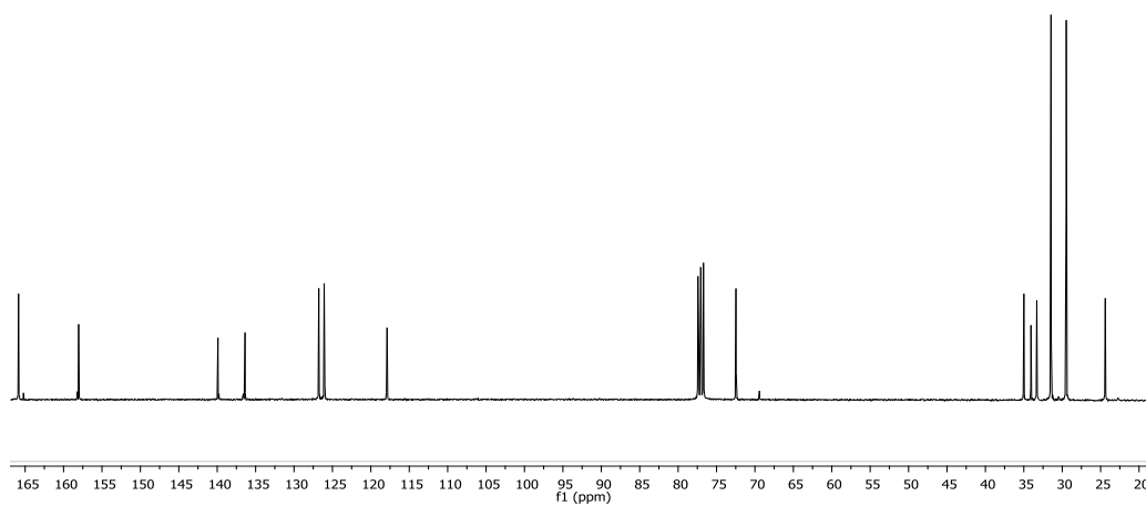
Espectro 8. Espectro de RMN ^{13}\text{C} (Tol-d8) para molécula
