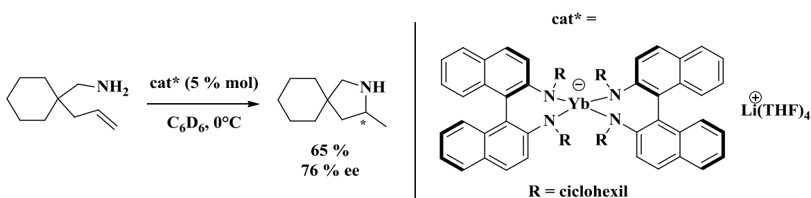
Esquema 23. Reacción de hidroaminación intramolecular.
