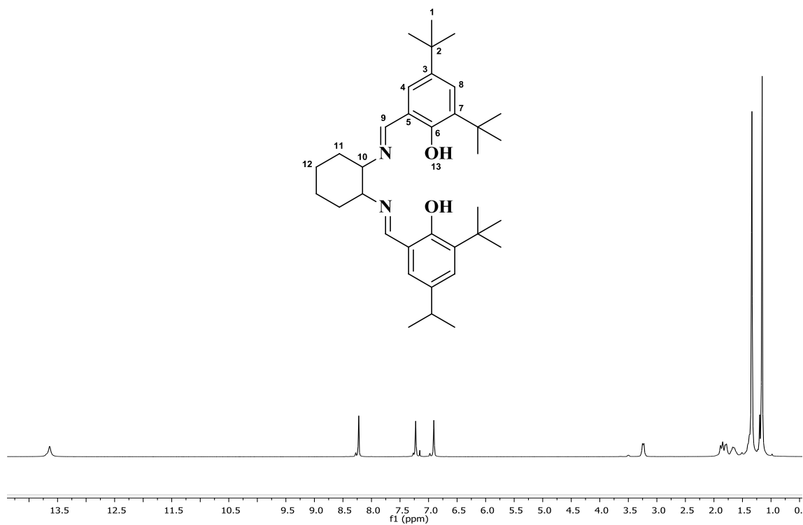
Espectro 7. Espectro de RMN ^1\text{H} (Tol-d8) para molécula 8.
