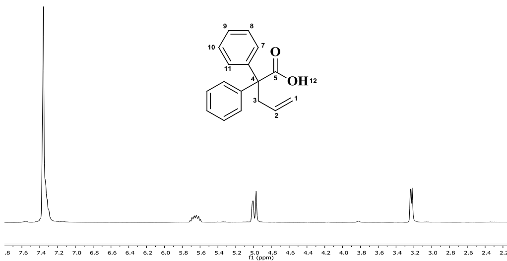
Espectro 11. Espectro de RMN 1 H (CDCl 3 ) para molécula 10.
