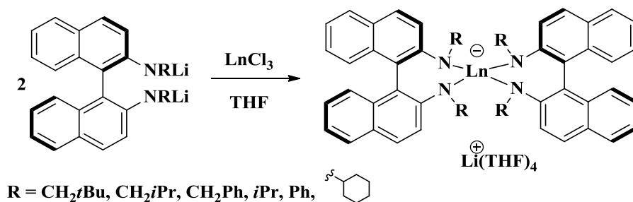
Esquema 22. Estructura general de complejo de binaftilamina.
