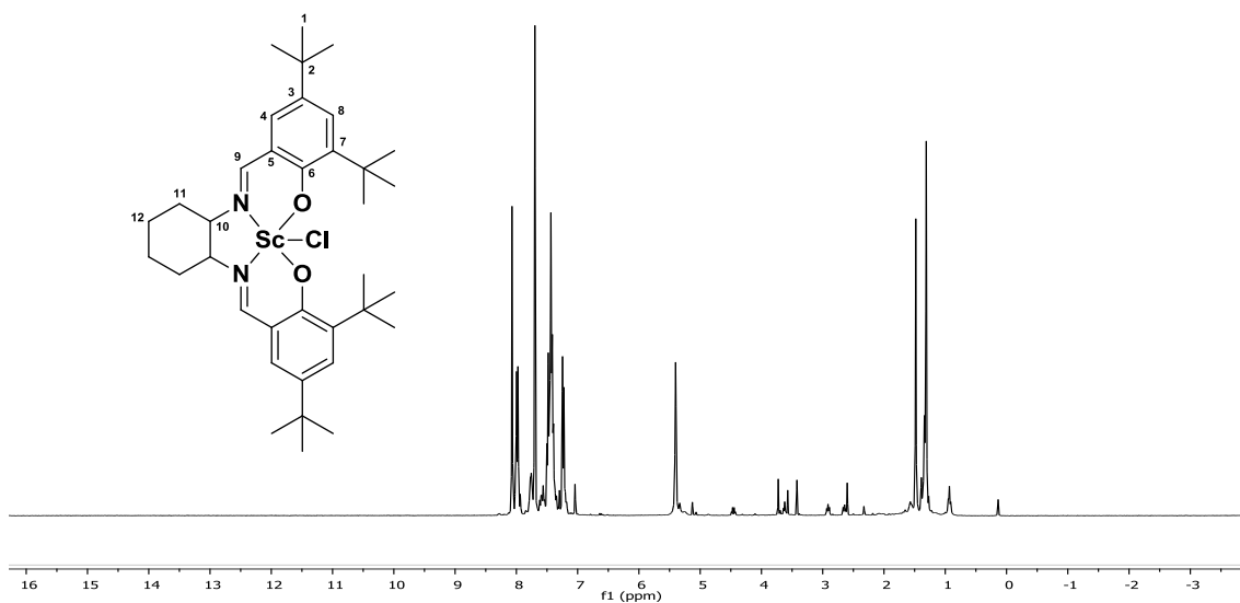
Espectro 11. Espectro de RMN 1 H (CDCl 3 ) para molécula 10.
