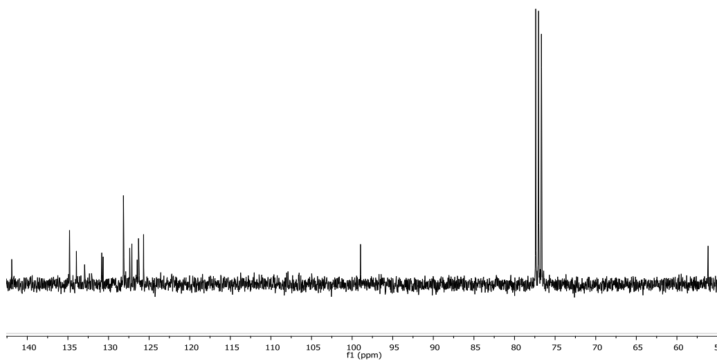
Espectro 6. Espectro de RMN ^{13}\text{C} ( \text{CDCl}_3 ) para molécula 4
