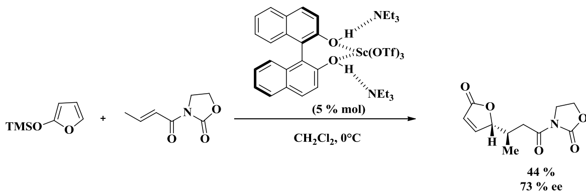
Esquema 4. Reacción de Michael.
