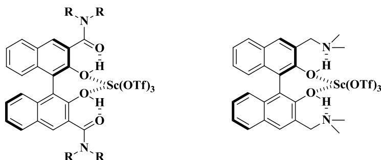
Esquema 5. Complejos de Katsuki.
