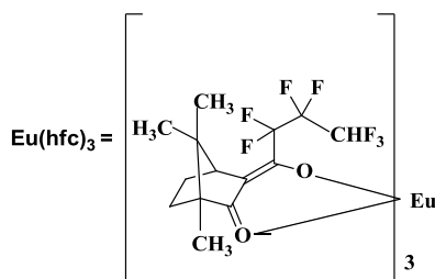
Esquema 2. Síntesis de dihidropironas utilizando Eu (hfc) 3 .
