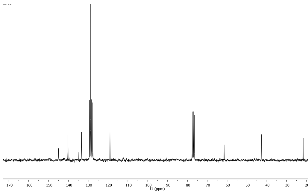
Espectro 14. Espectro de RMN ^{13}\text{C} ( \text{CDCl}_3 ) para molécula 11.
