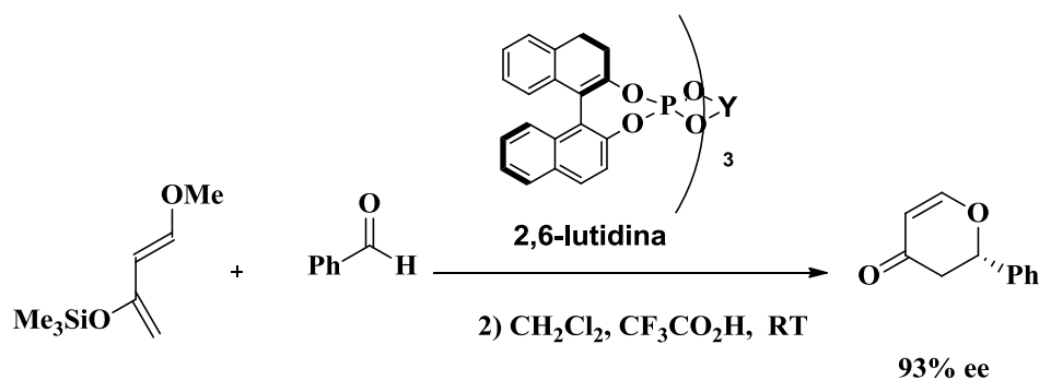
Esquema 18. Reacción de Diels-Alder.
