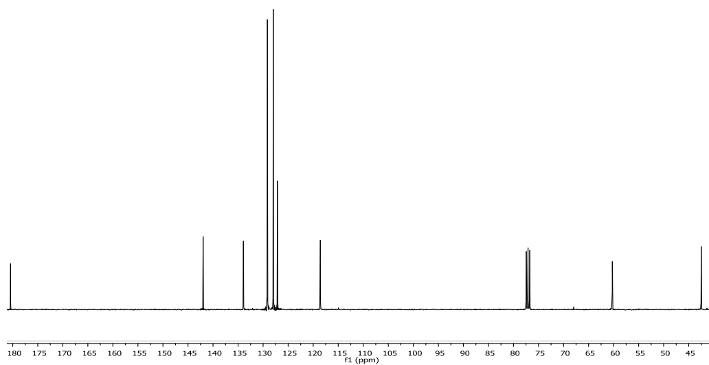
Espectro 12. Espectro de RMN ^{13}\text{C} ( \text{CDCl}_3 ) para molécula 10
