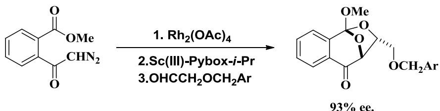
Esquema 8. Reacción de cicloadición de Suga.
