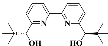
Esquema 12. Ligante de Bolm.
