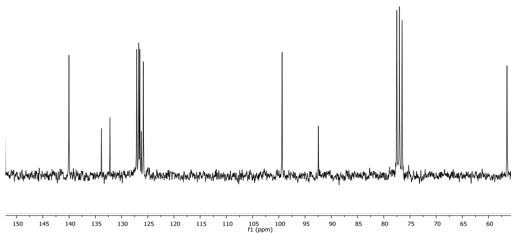
Espectro 4. Espectro de RMN ^{13}\text{C} ( \text{CDCl}_3 ) para molécula 3.
