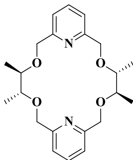
Esquema 11. Ligante poliheteroatómico de Kobayashi.
