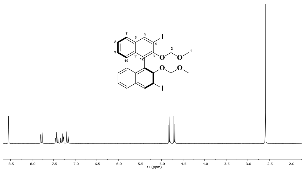
Espectro 3. Espectro de RMN ^1\text{H} ( \text{CDCl}_3 ) para molécula 3
