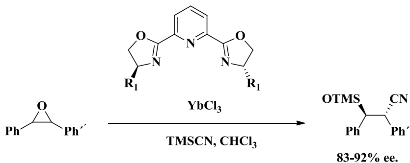
Esquema 9. Apertura de epóxidos de Jacobsen.
