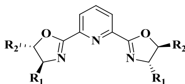
Esquema 7. Estructura general del ligante Pybox.
