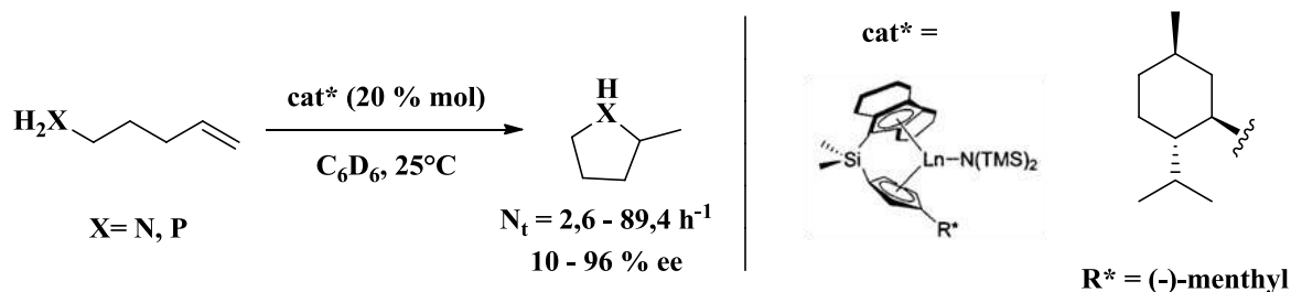
Esquema 15. Hidroaminación intramolecular.
