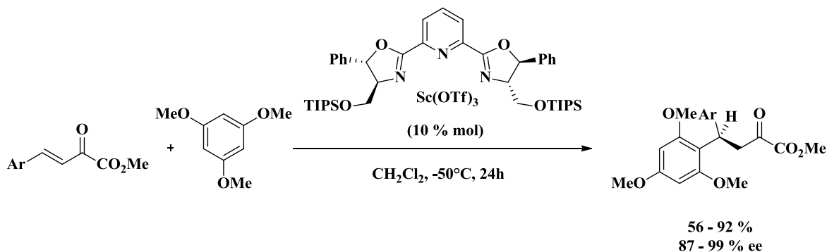
Esquema 10. Reacción de Friedel-Crafts de Evans.
