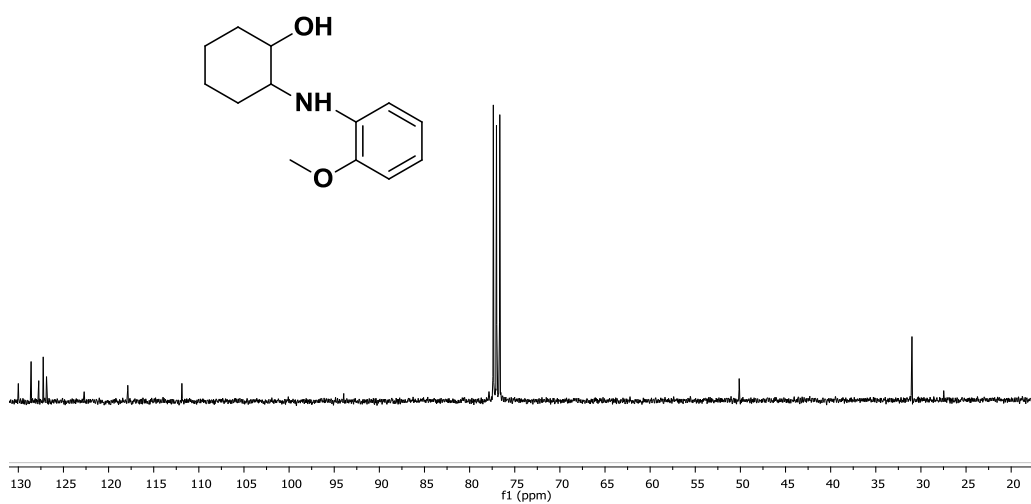
Espectro 15. Espectro de RMN ^{13}\text{C} ( \text{CDCl}_3 ) para molécula 12.
