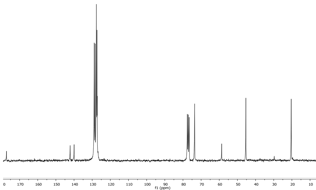
Espectro 17. Espectro de RMN ^{13}\text{C} (Tol-d8) para molécula 13
