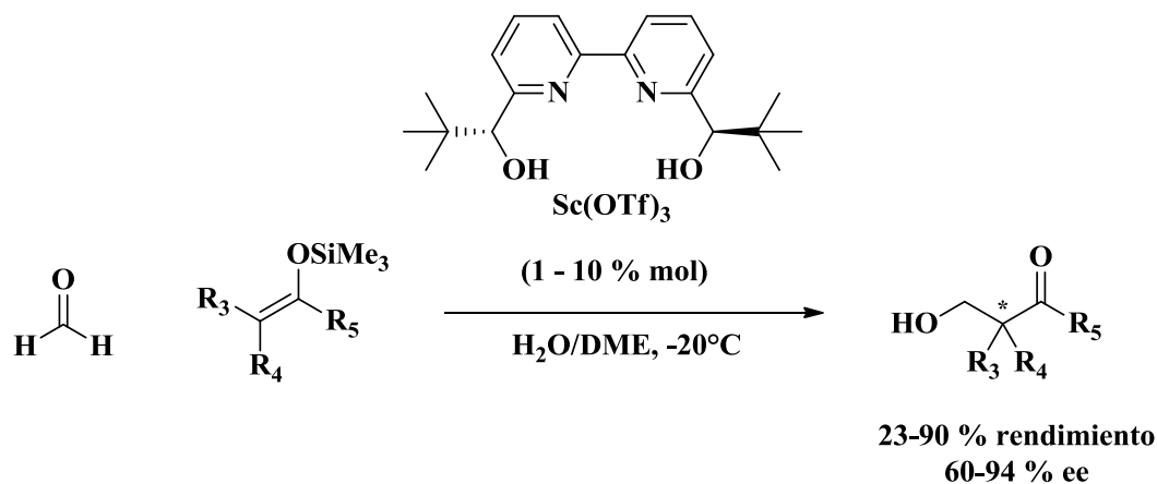
Esquema 13. Reacciones de hidroximetilación de Kobayashi.
