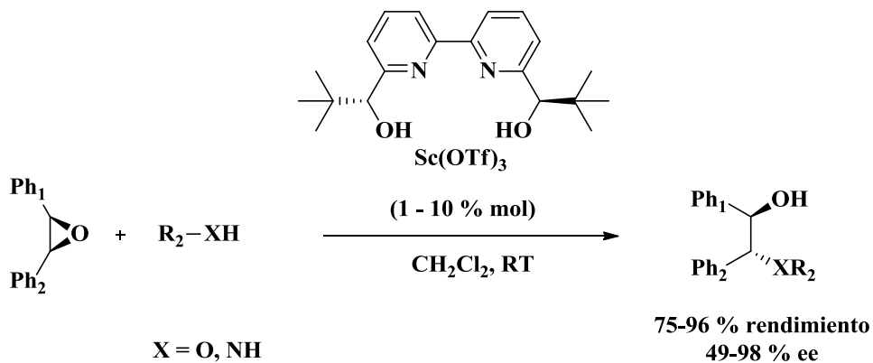
Esquema 14. Apertura de epóxidos de Schneider.
