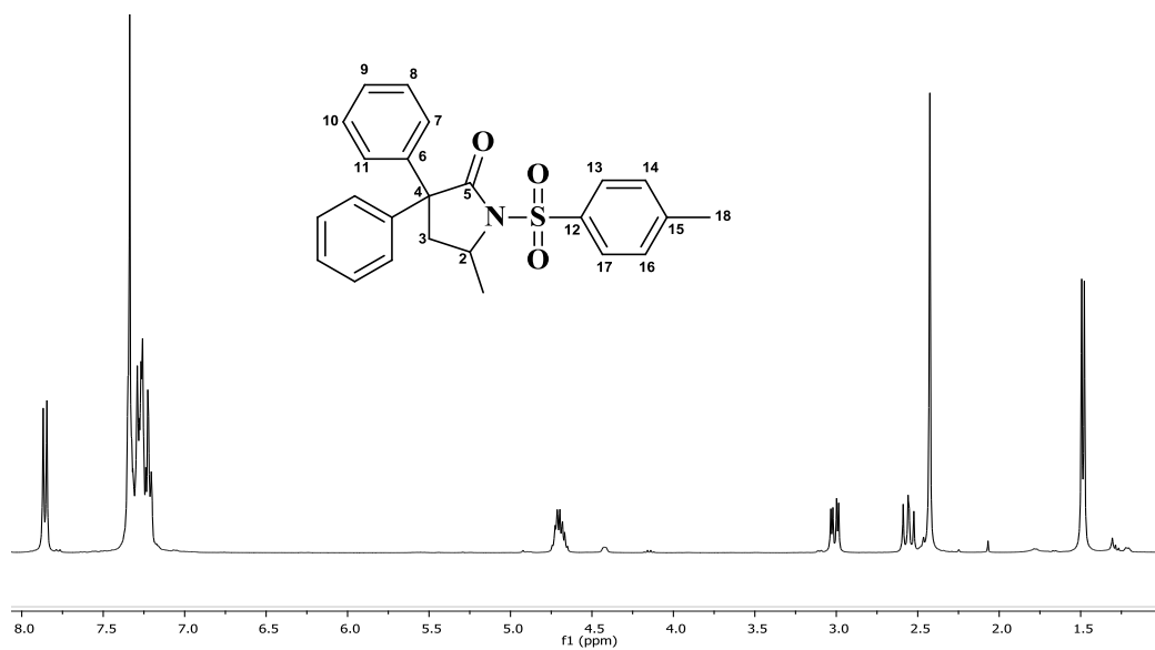
Espectro 18. Espectro de RMN ^1\text{H} (Tol-d8) para molécula 14
