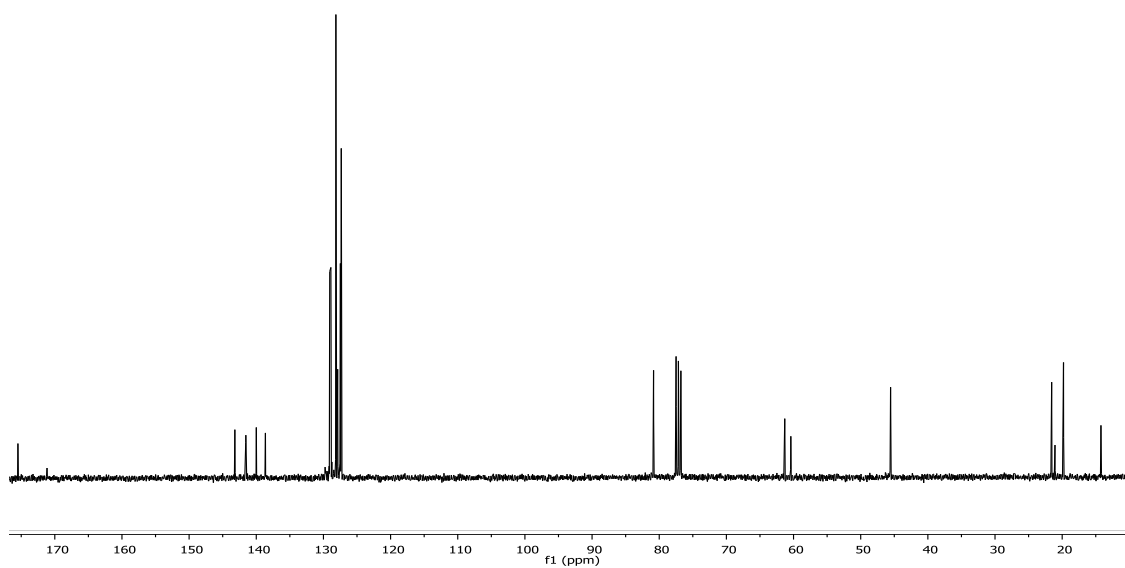
Espectro 19. Espectro de RMN ^{13}\text{C} (Tol-d8) para molécula 14
