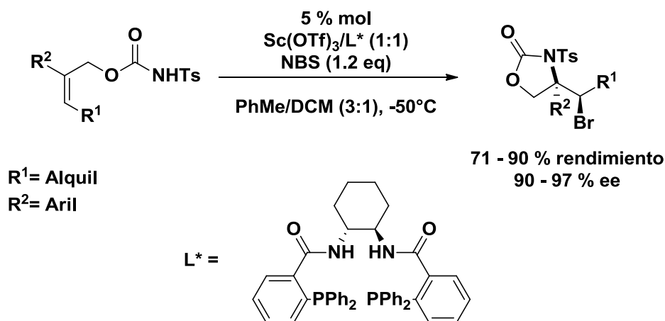
Esquema 6. Bromoaminociclización de N -tosilcarbamatos de alilo.
