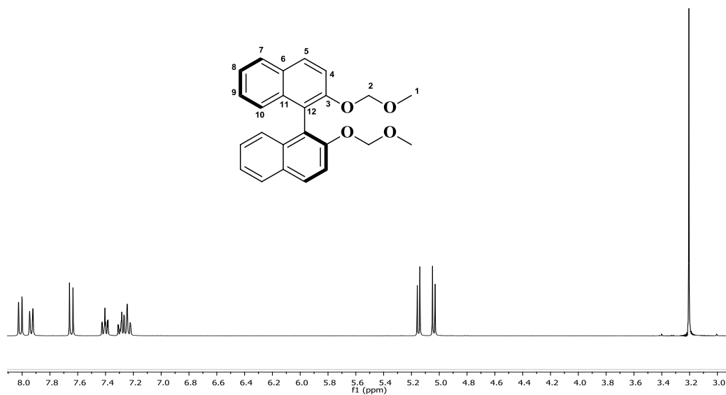
Espectro 1. Espectro de RMN 1 H (CDCl 3 ) de molécula 2
