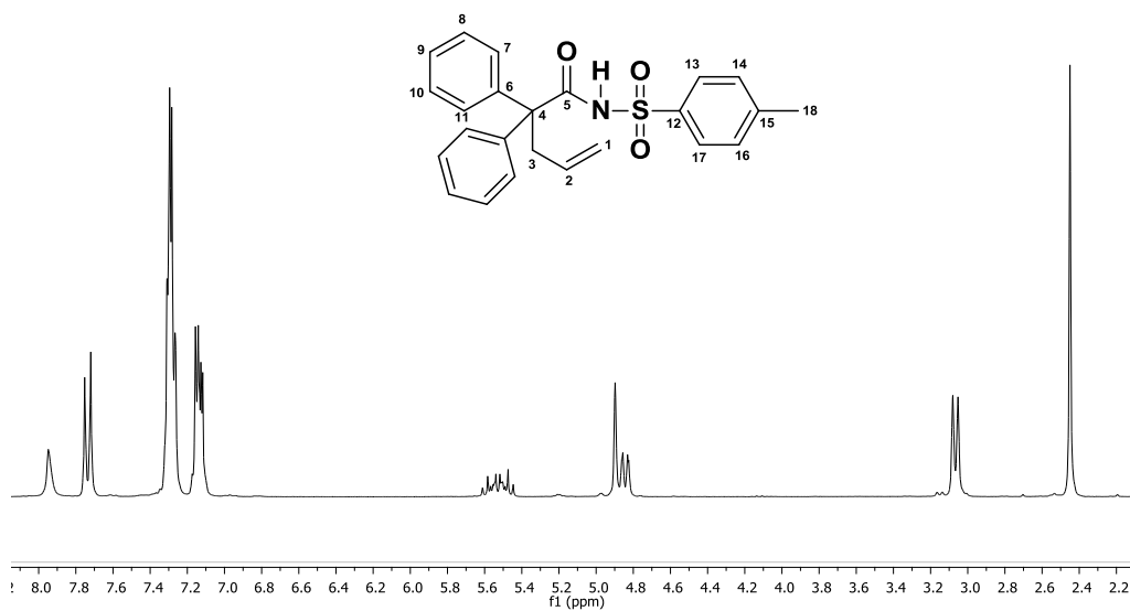
Espectro 13. Espectro de RMN ^1\text{H} ( \text{CDCl}_3 ) para molécula 11.
