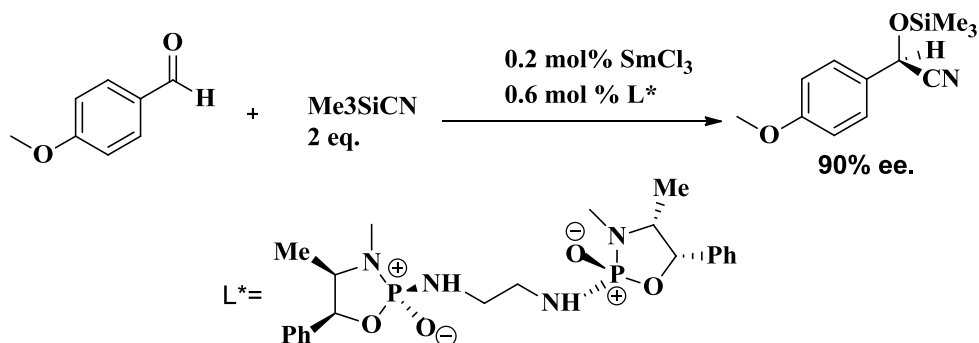
Esquema 19. Reacción de cianosililación de aldehídos de Fang.
